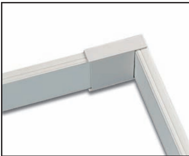
ÁNGULO EXTERIOR: Troquele las paredes A y D OUTER ANGLE: Cut out walls A and D
