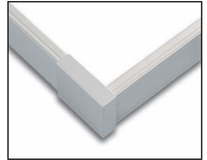
ÁNGULO INTERIOR: Utilice el accesorio sin troquelar INNER ANGLE: Use the accessory directly
